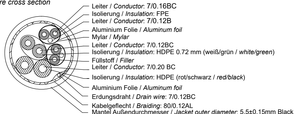
Aderquerschnitt / Wire cross section
