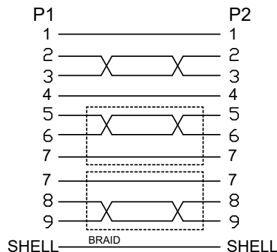
Anschlussdiagramm / Wiring diagram
