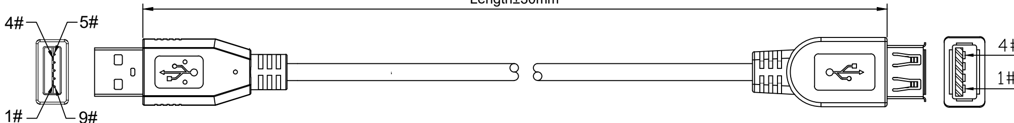
Anschlussdiagramm / Wiring diagram
